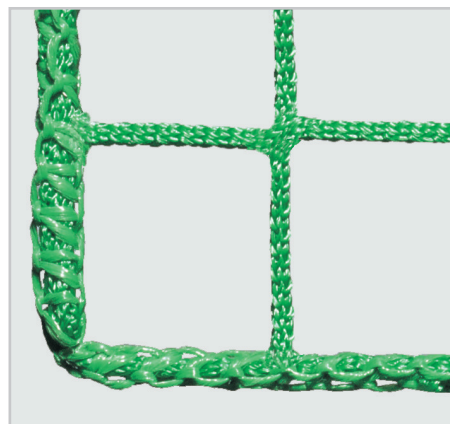
obšití lemu sítě 5 - 7 mm
